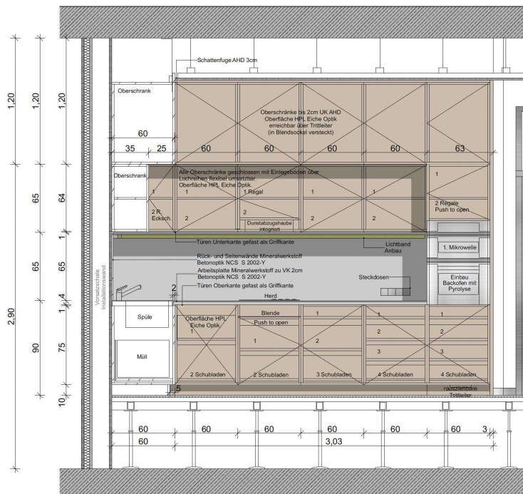
SCHNITTANSICHT M1:20
